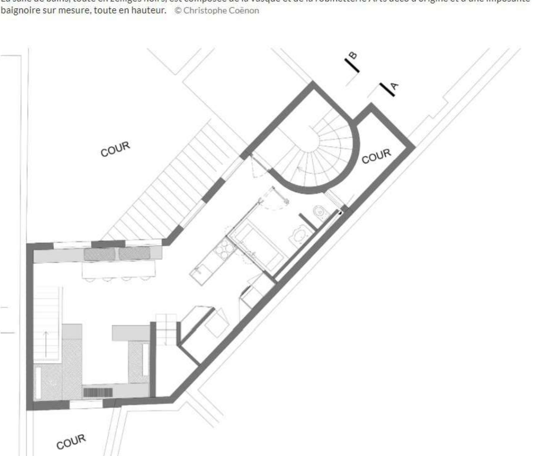
Le plan de l'appartement après les travaux.
